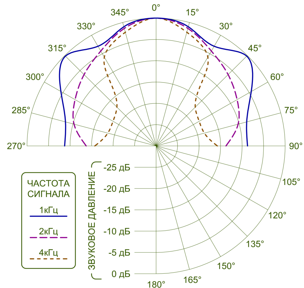
Рис.1 Характеристика направленности прожектора звукового МЕТА 7663 .
